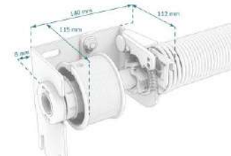
Détails Ressorts Avant :
