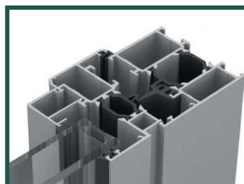
Profilé avec rupture de pont thermique
