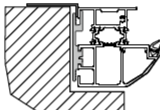
Solution pour pose en feuillure (suppression de l'huissérie existante)
