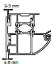
Huissérie en aluminium avec bride de fixation
