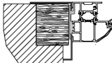
Solution pour pose sur huissérie bois existante
