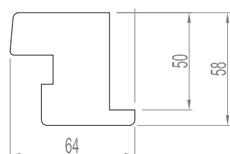
Dormant rénovation
