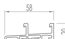
Seuil
