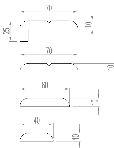
Habillage bois
