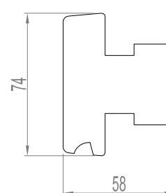
Traverse intermédiaire
