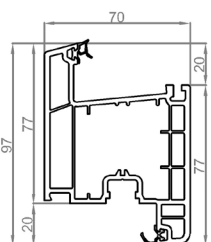
Profil ouvrant porte service ou porte cintrée
