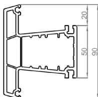
Montant et traverse intermédiaire dormant
