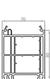
Elargisseurs (pour dormant carré)
