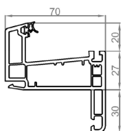
Dormant à recouvrement
